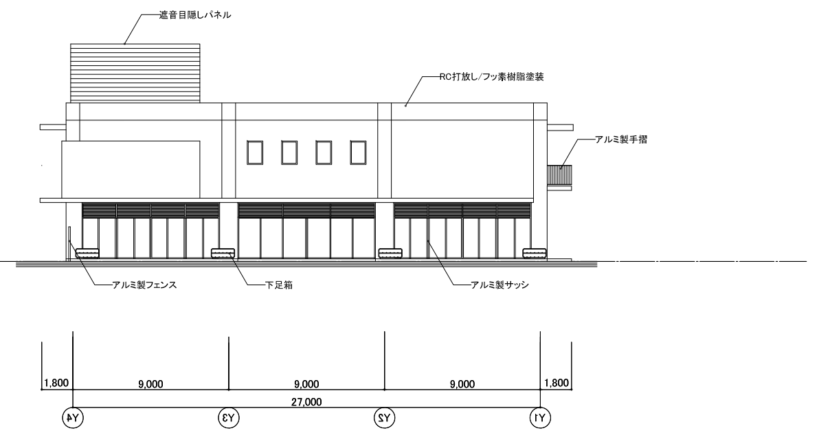
西側立面図
