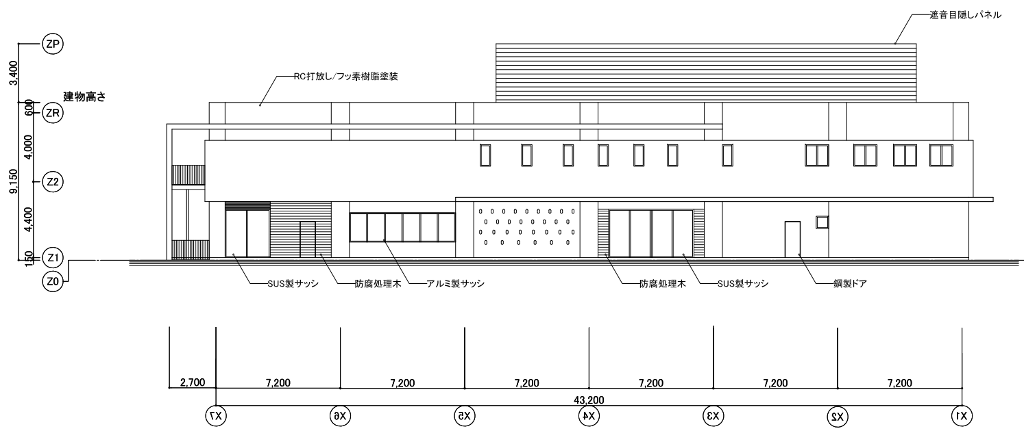
北側立面図
