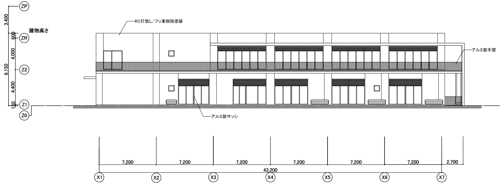
南側立面図
