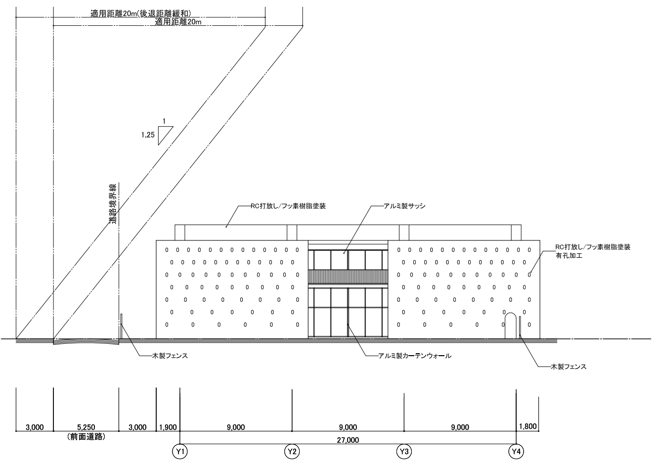
東側立面図
