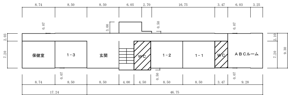
1 階 平 面 図
