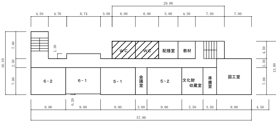
3 階 平 面 図
