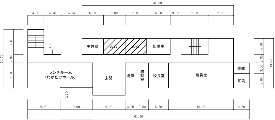
1 階 平 面 図
