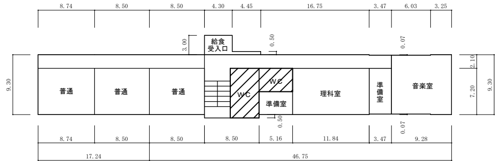
3 階 平 面 図
