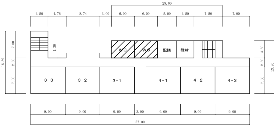
4 階 平 面 図
