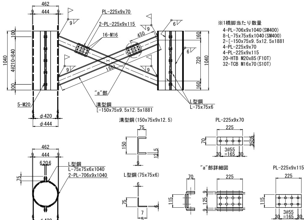
ブレース材詳細図 S=1:20
