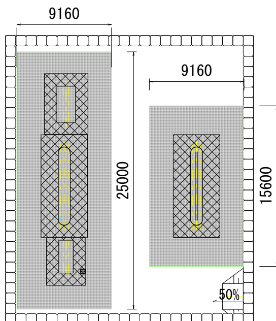
図-2 掘削範囲
