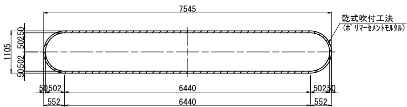
平面図 ( 1 - 1 )
