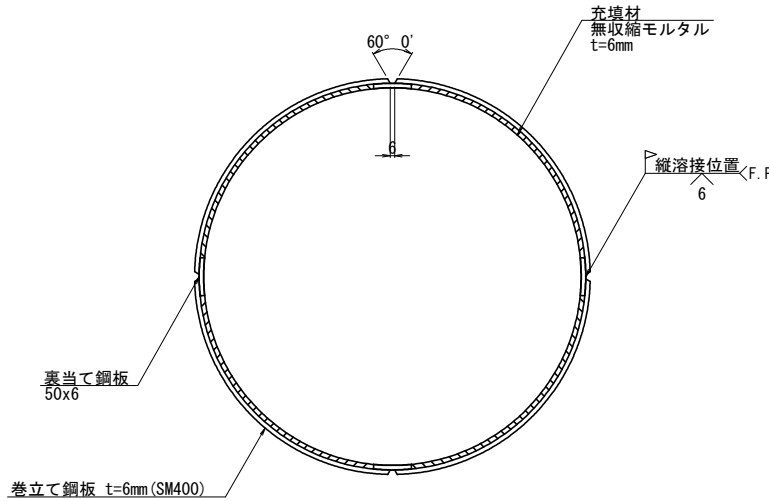
ブレース材詳細図 S=1:20
