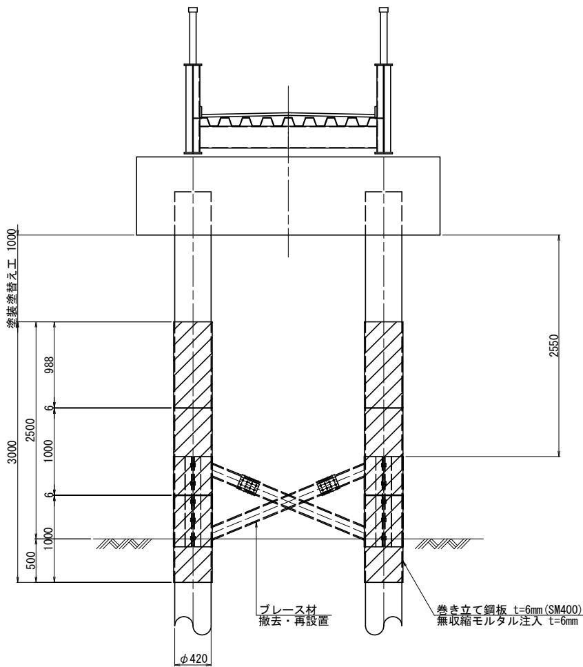
正面図 S=1:30
