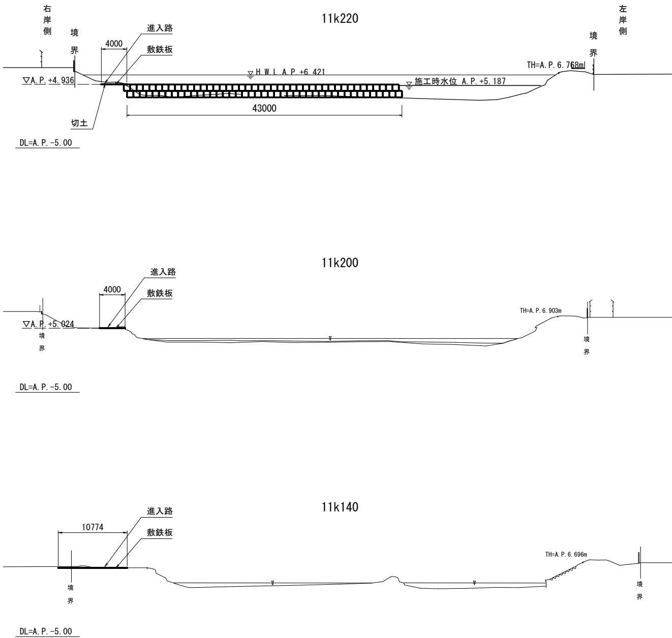
横断図
