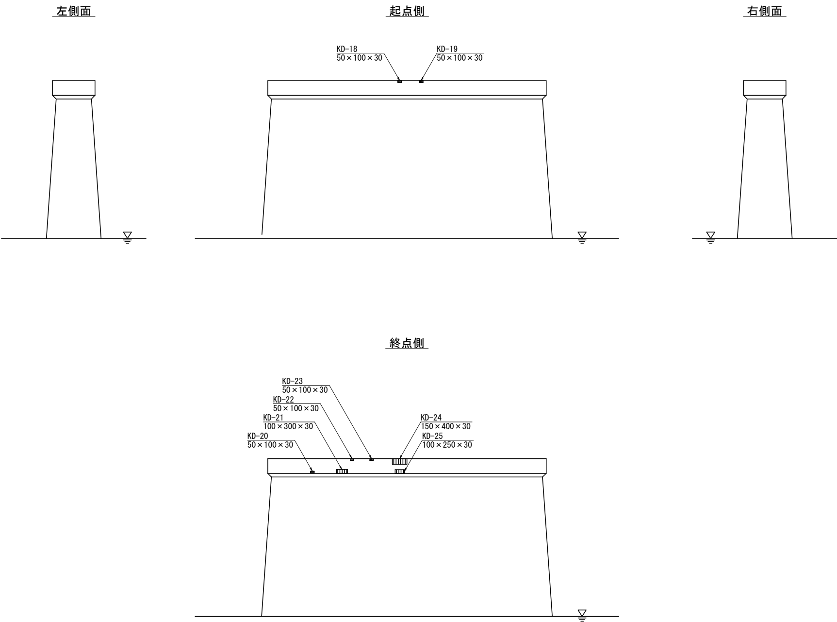
P3橋脚
