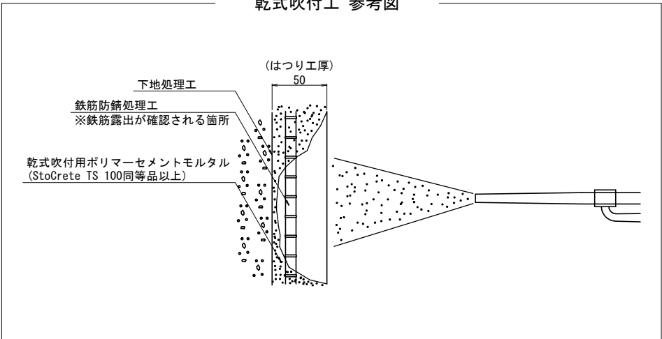
乾式吹付工 参考図
