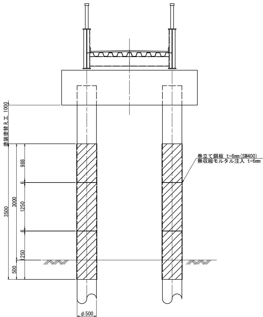
正面図 S=1:30
