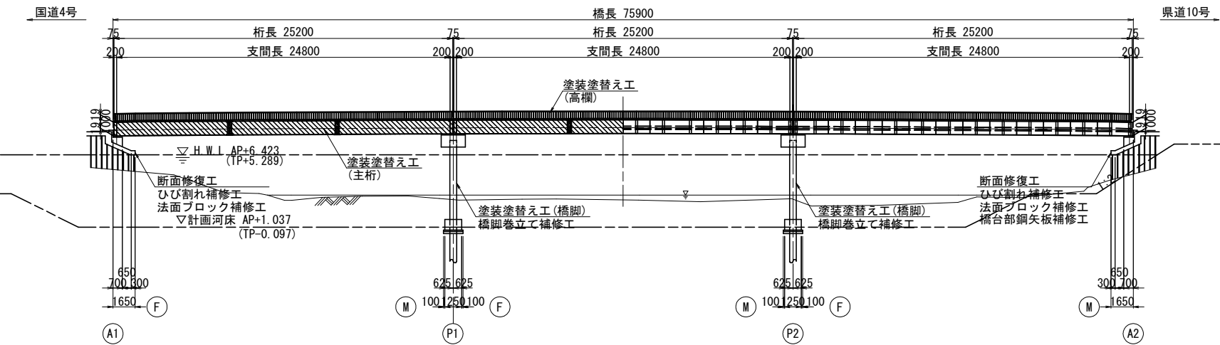
側面図(下流側) S=1:200
