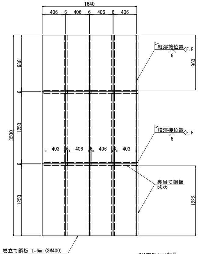
巻立て鋼板加工図 S=1:20
