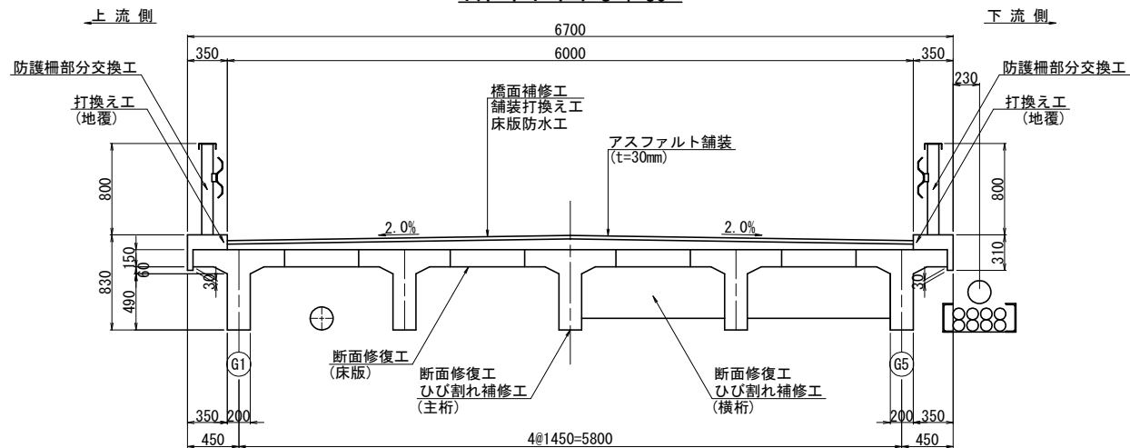
断面図 S=1:30
