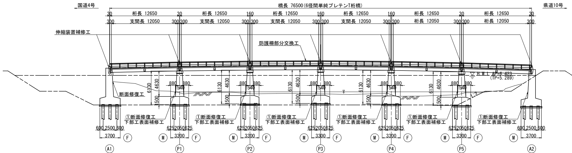
側面図 S=1:200
