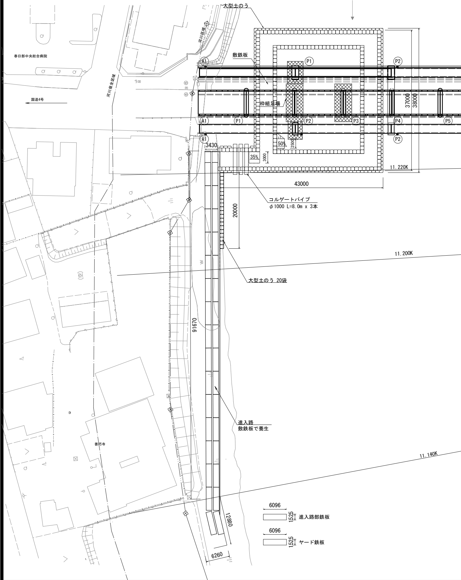
平面図
