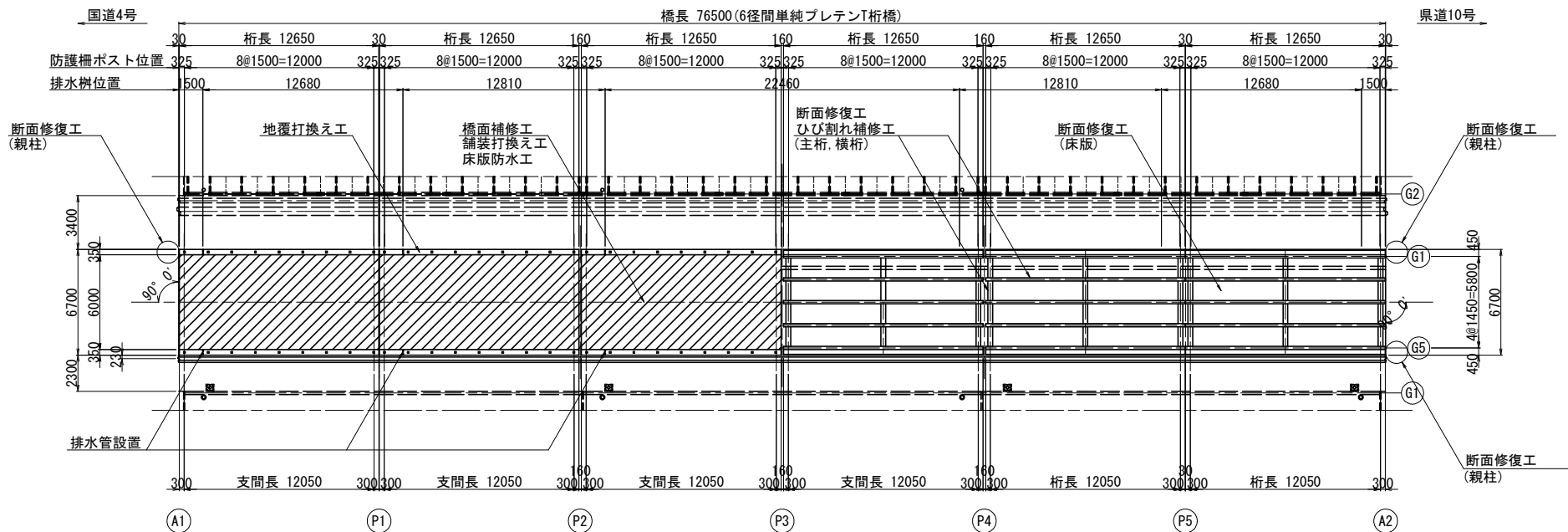
平面図 S=1:200
