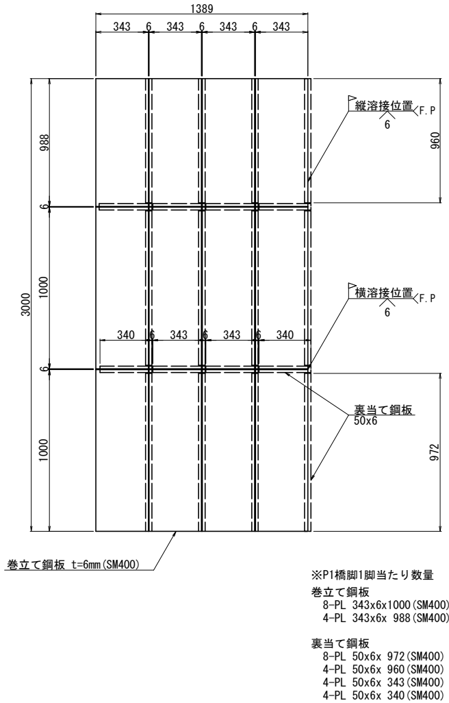
巻立て鋼板加工図 S=1:20
