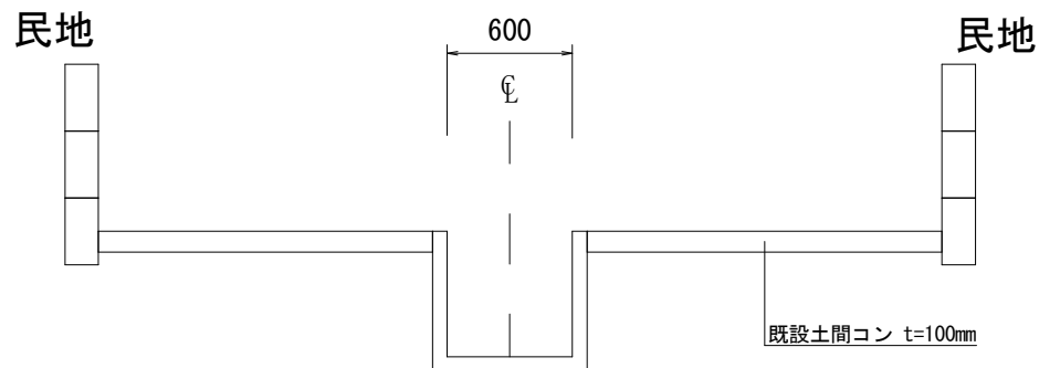
現況断面図
