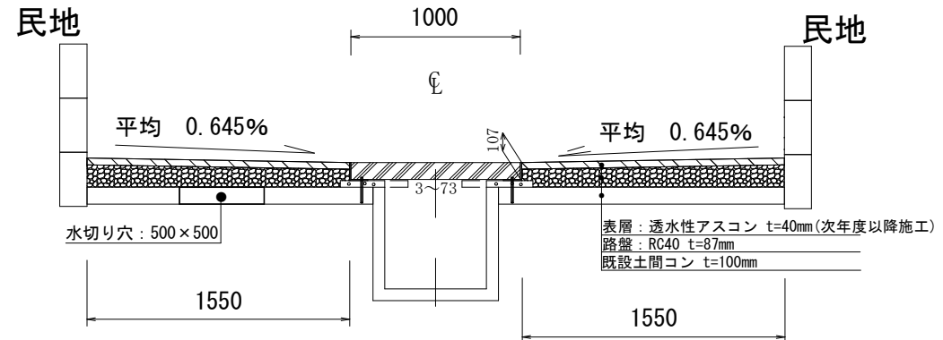
計画断面図
