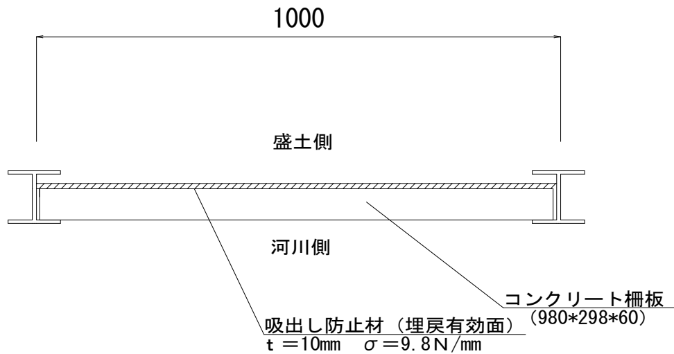
平面図 S=1 : 10
