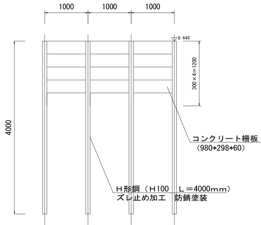
側面図 S=1 : 50
