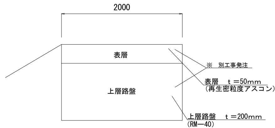
路盤組成図 S=Free
