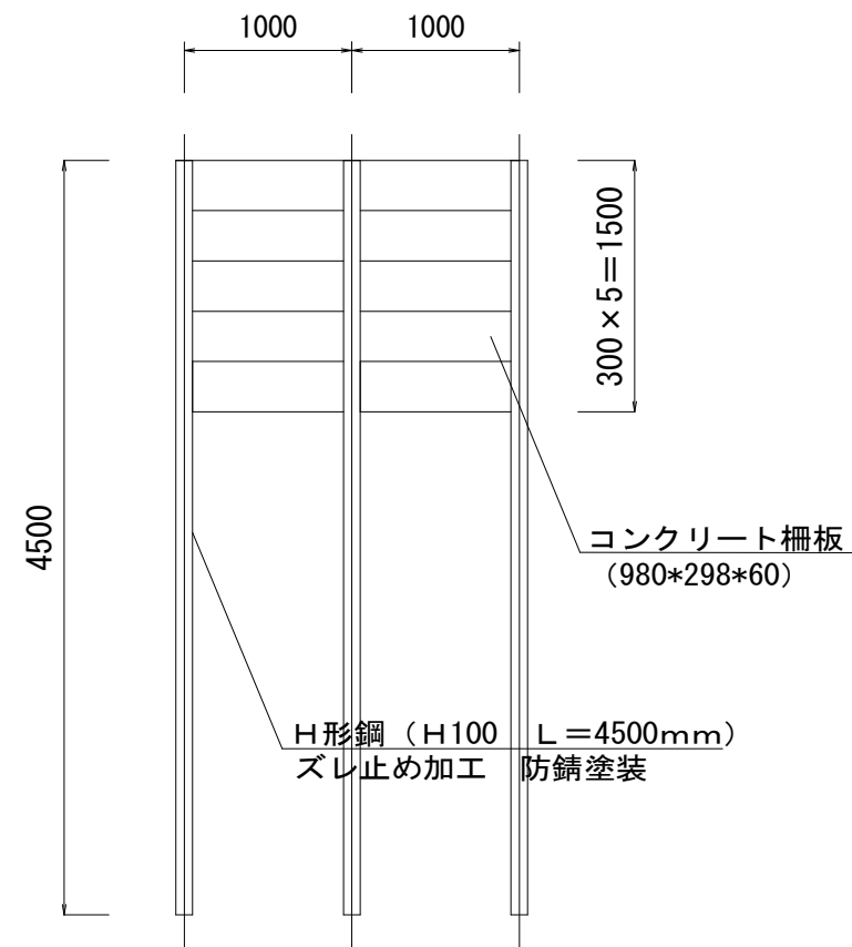
側面図 S=1 : 50
