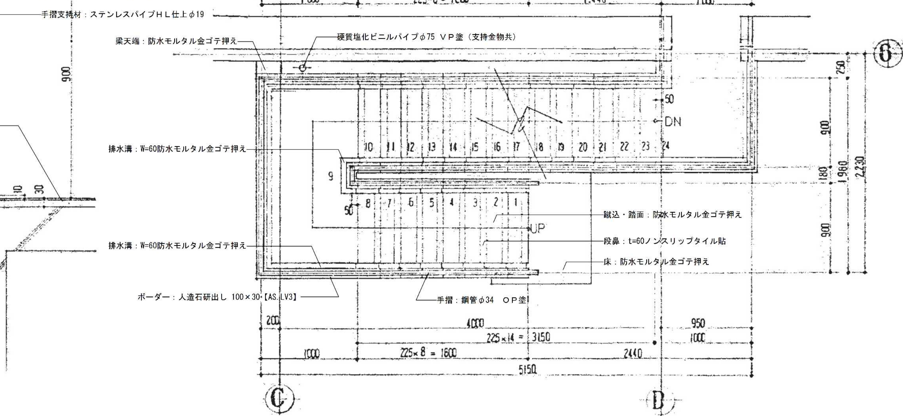
屋外階段 平面詳細図 S=1/25
