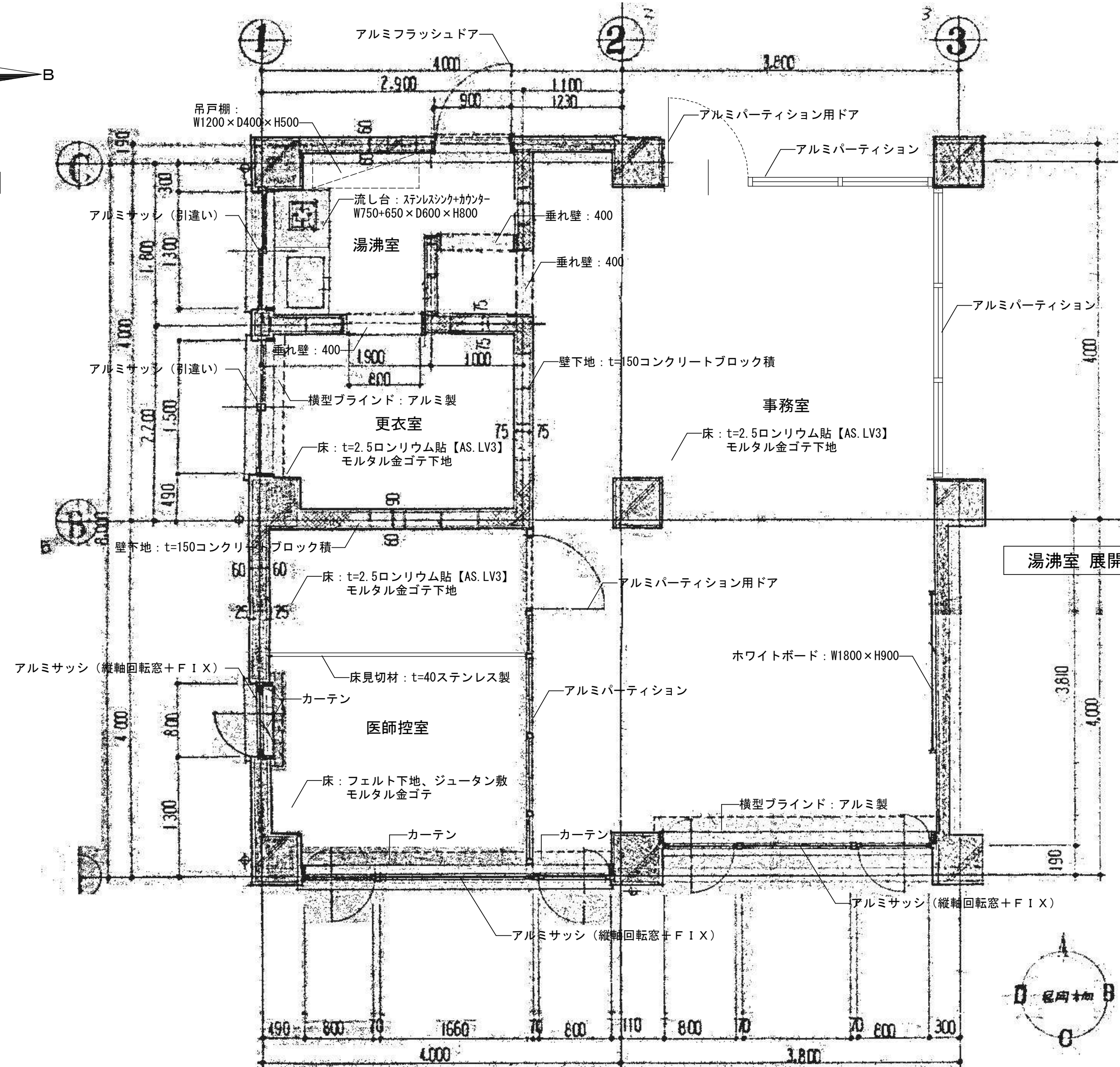
事務室廻り 平面詳細図 S=1/40
