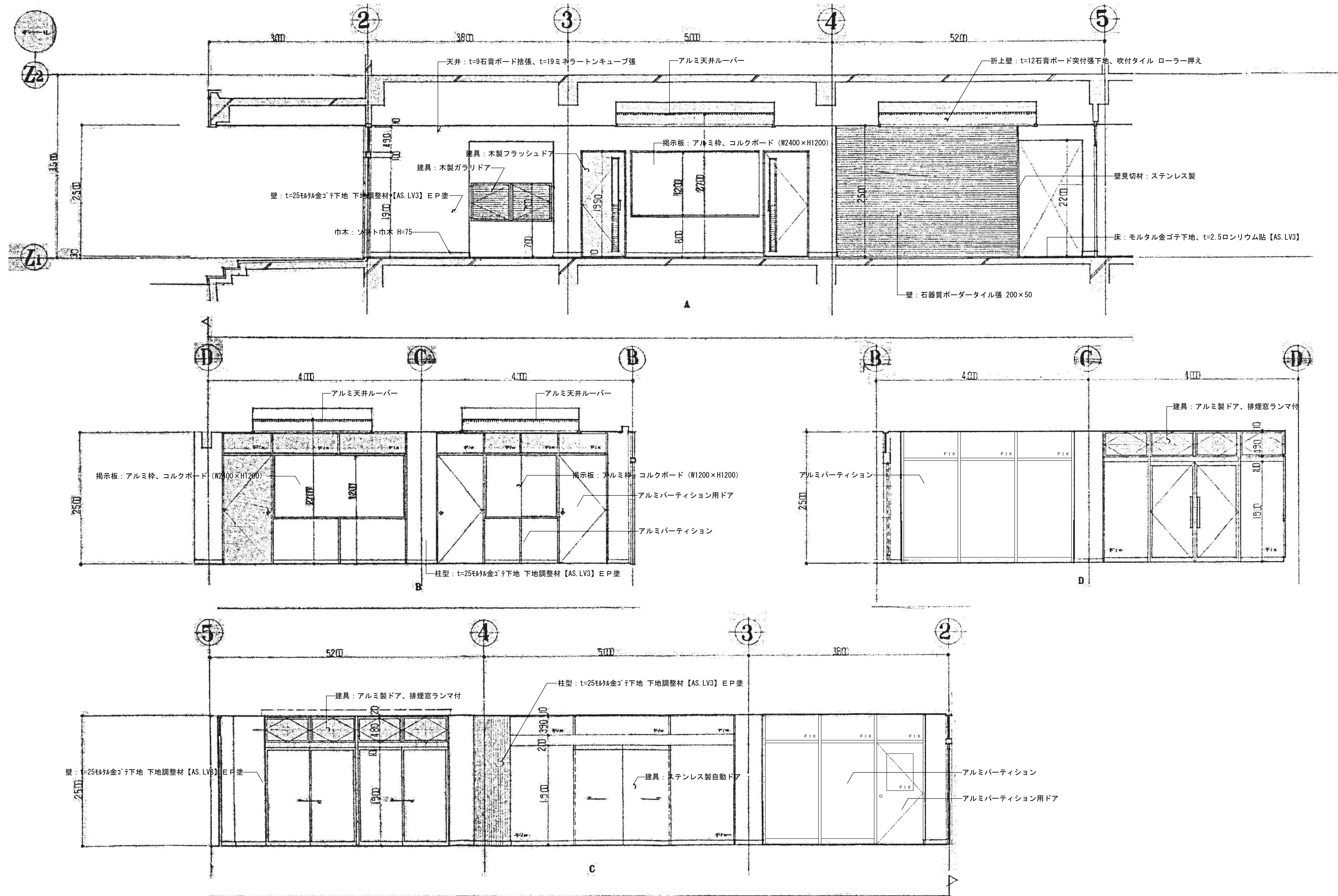
ホール 展開図 S=1/40
