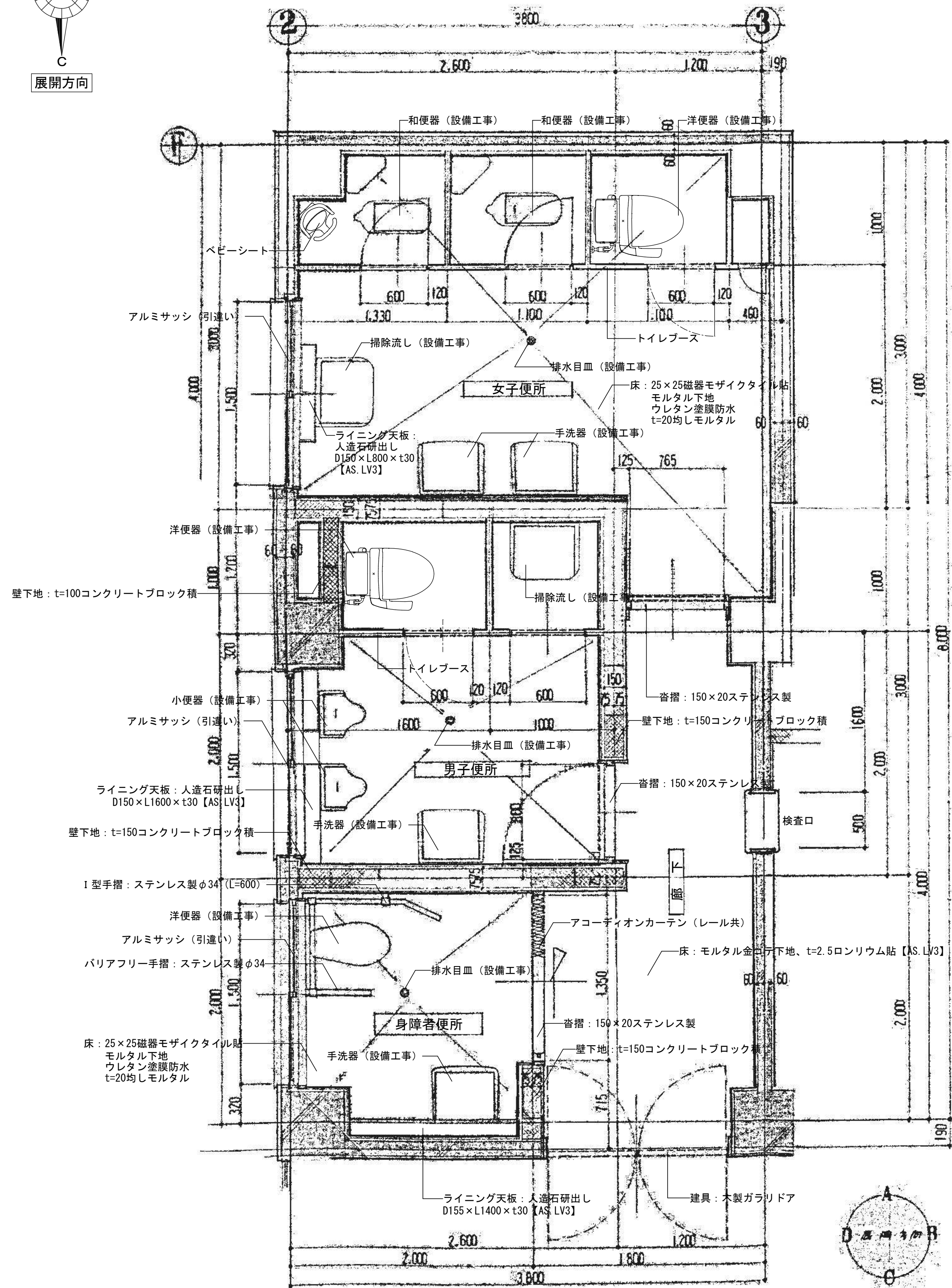
1階便所廻り 平面詳細図 S=1/25
