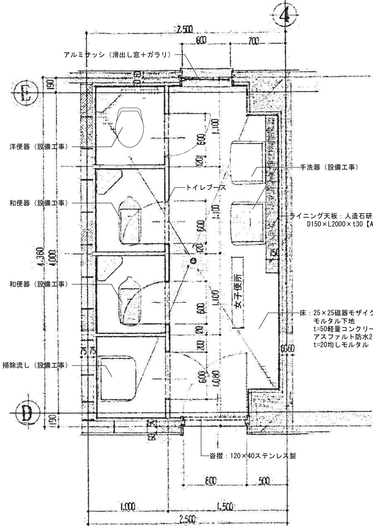
2階便所廻り 平面詳細図 S=1/25
