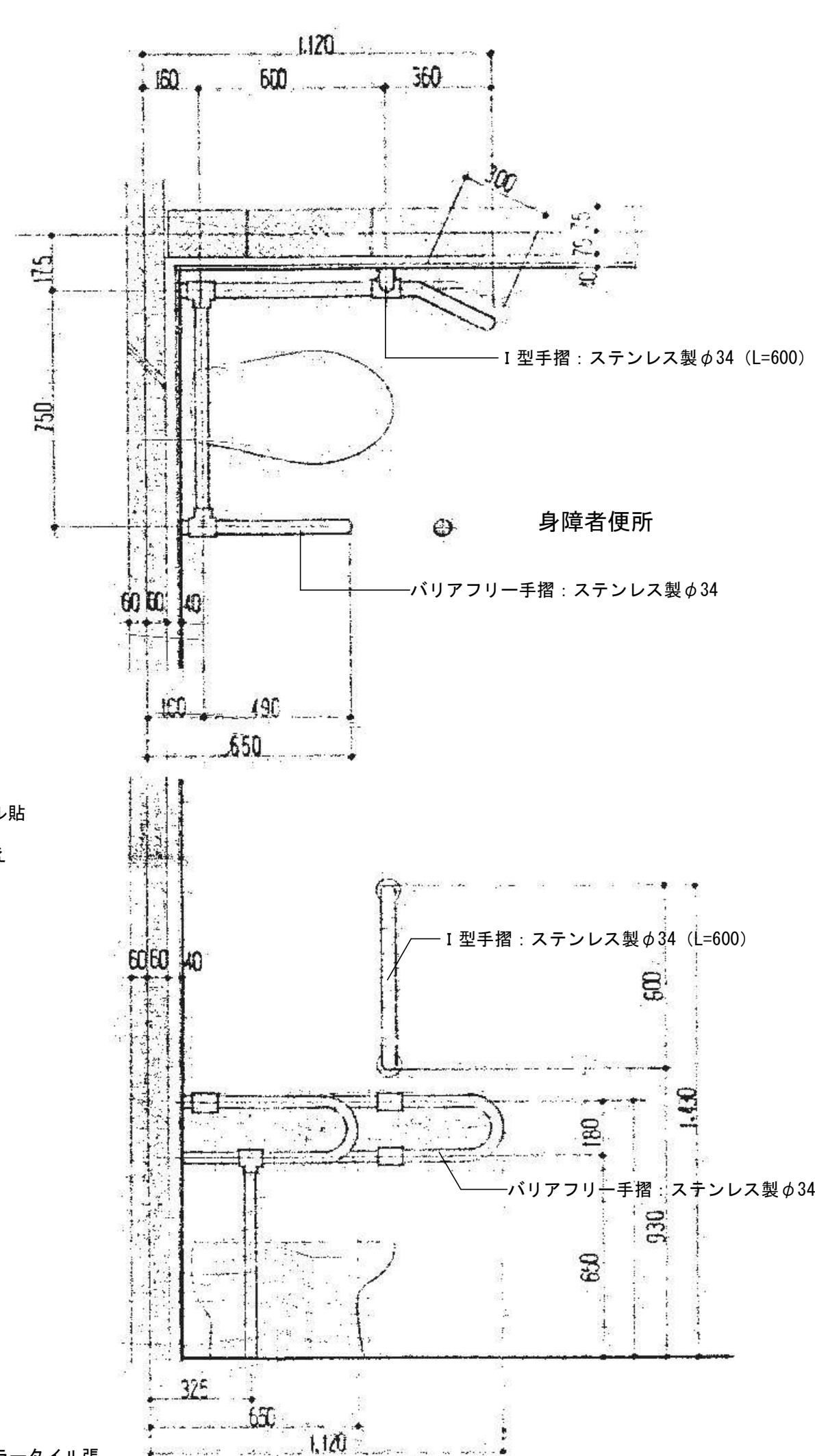
身障者用手摺詳細図 S=1/15
