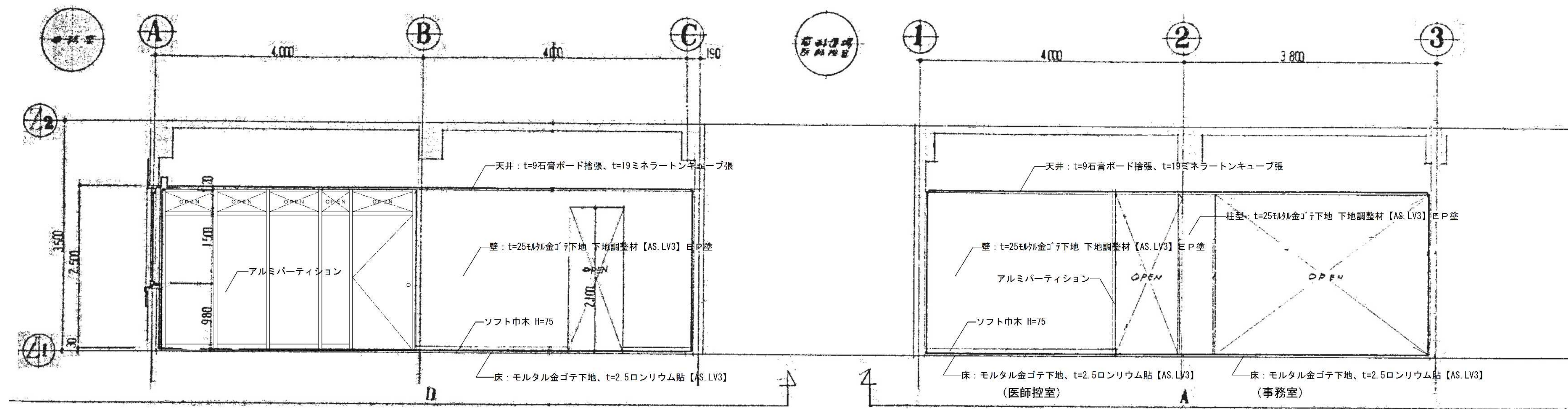
事務室 展開図 S=1/40
