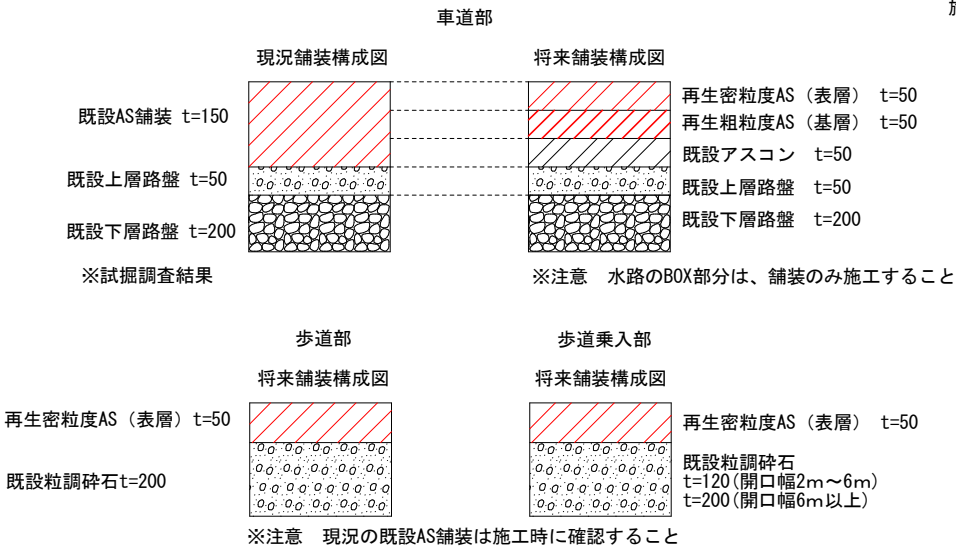
舗装構成図 S=Free
