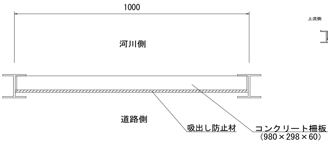
平面図
