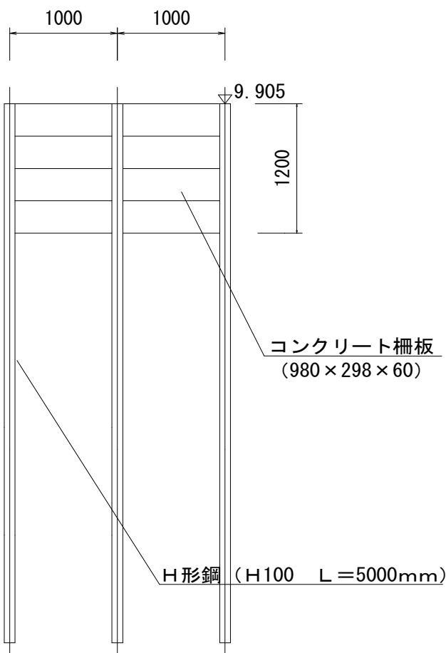
側面図 S=1:50
