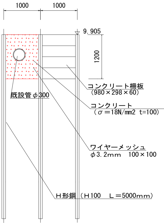
現場打側面図 S=1:50
