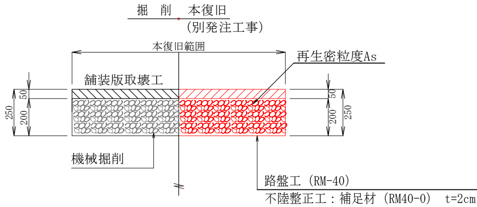
路盤組成図 S=Free
