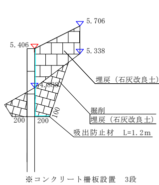
断面図 S=1 : 5 0
