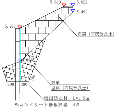
断面図 S=1 : 5 0
