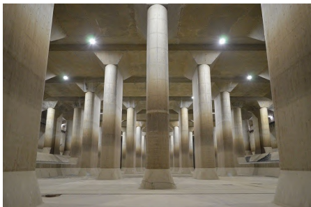
首都圏外郭放水路
