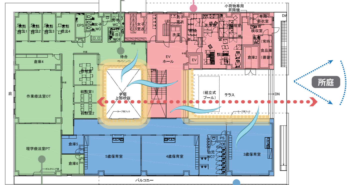
2階平面図
