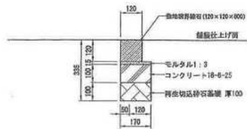
景地境界線石 (SE-1) 詳細図 S=1/10
