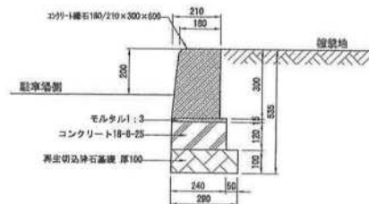
歩車道境界線石 (E-2) 詳細図 S=1/10
