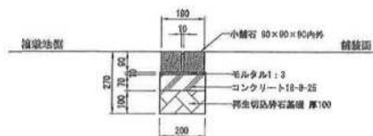
小舗石線石 (SH) 詳細図 S=1/10
