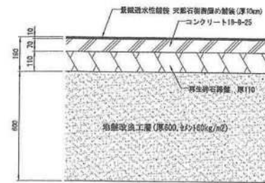
交流広場舗装 (景観透水性舗装部) 標準断面図 S=1/10
