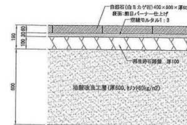
交流広場舗装 (自然石部) 標準断面図 S=1/10
