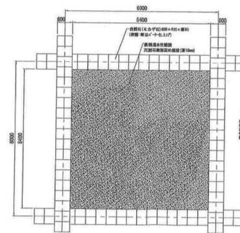
交流広場舗装工基本グリット平面図 S=1/40
