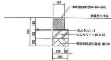
景地境界線石 (SE-2) 詳細図 S=1/10
