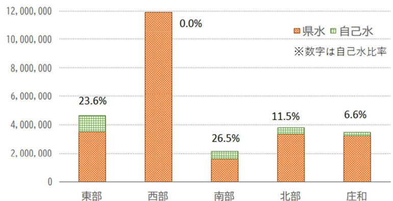
図表3 令和4年度 各浄水場の原水量および比率グラフ
