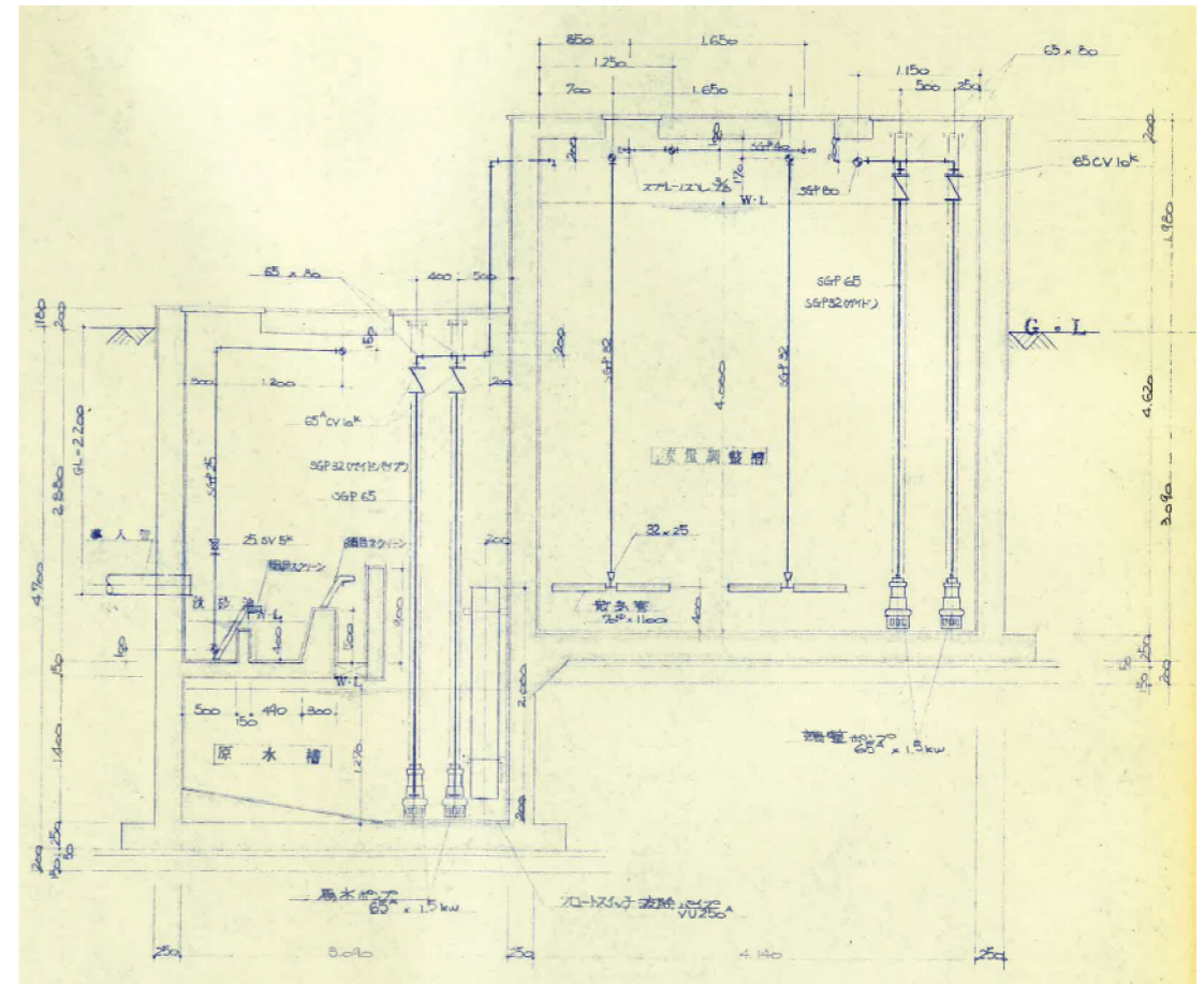
合併処理浄化槽断面図④(参考図) : Non Scale
