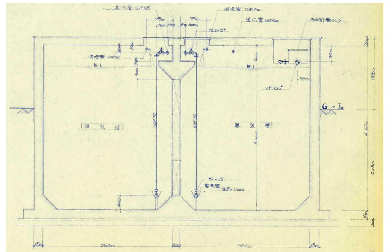
合併処理浄化槽断面図④(参考図) : Non Scale
