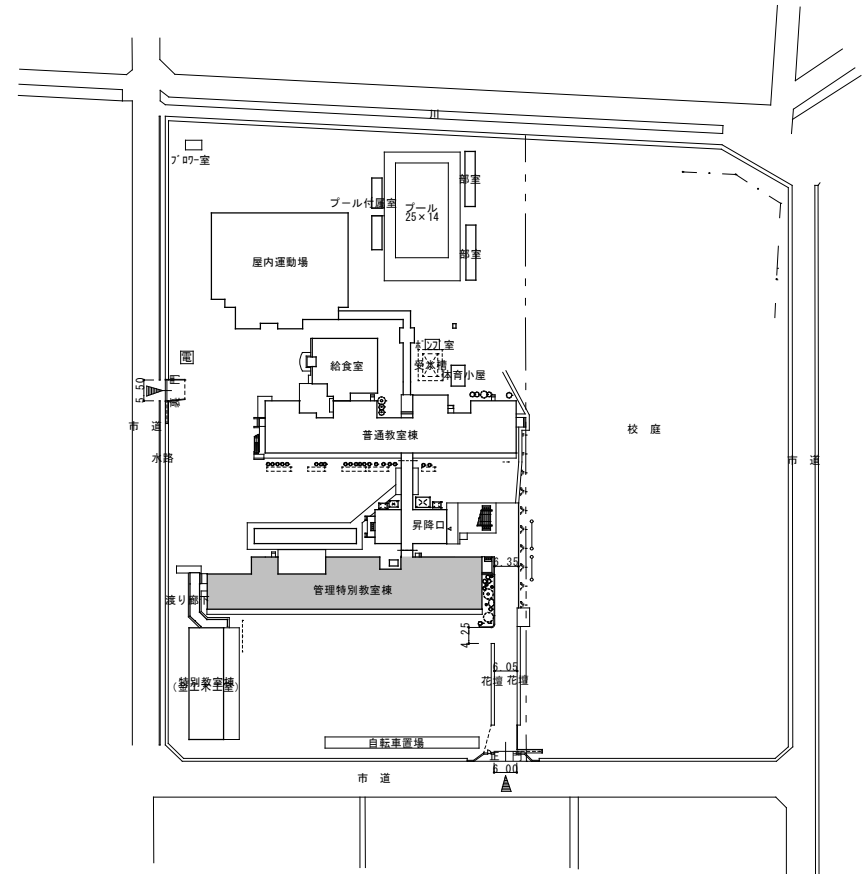
配置図
